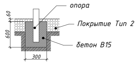
Узел установки опоры
